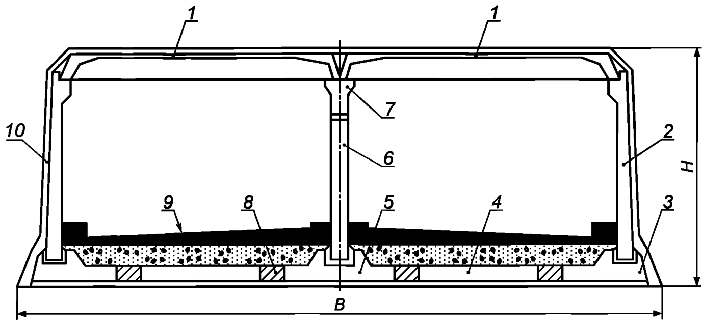
H — высота по оси тоннеля; B — ширина тоннеля; 1 — блок перекрытия; 2 — стеновой блок; 3 — фундаментный блок; 4 — лотковый блок; 5 — подколونник; 6 — колонна; 7 — прогон; 8 — омоноличивающая обвязка стыков блоков; 9 — проезжая часть; 10 — гидроизоляция
