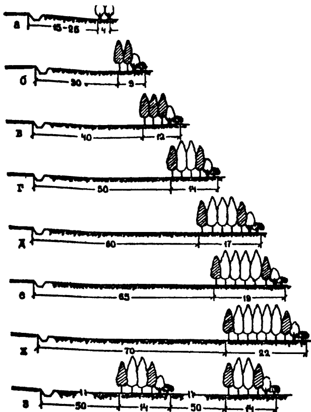
Рис. 3.1. Типовые схемы снегозащитных лесных насаждений вдоль автомобильных дорог при объеме снегопереноса ( m^3/m ).
