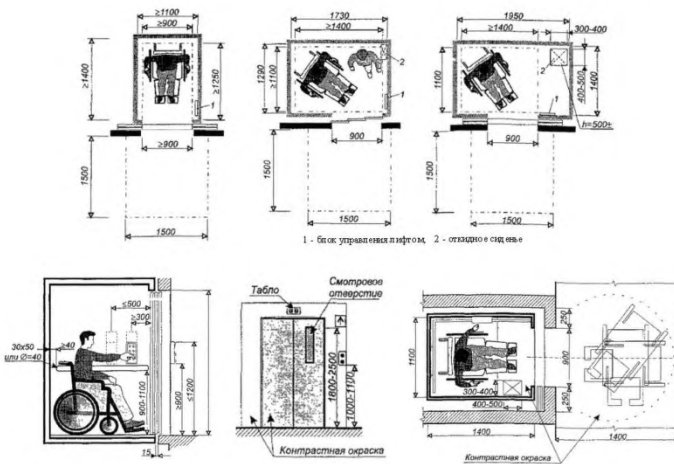
Рисунок 17– Основные параметры лифта для инвалидов и других маломобильных групп населения
