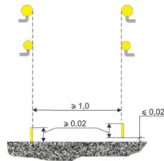
Рисунок 14– Параметры размещения бортиков безопасности
