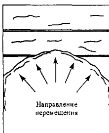
Рисунок 43 – Строительство насыпи с U-образным перемещением
