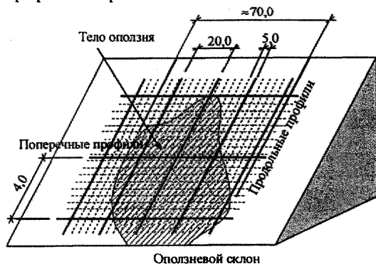
Рисунок В.2 – Схема расположения профилей на оползневом склоне
