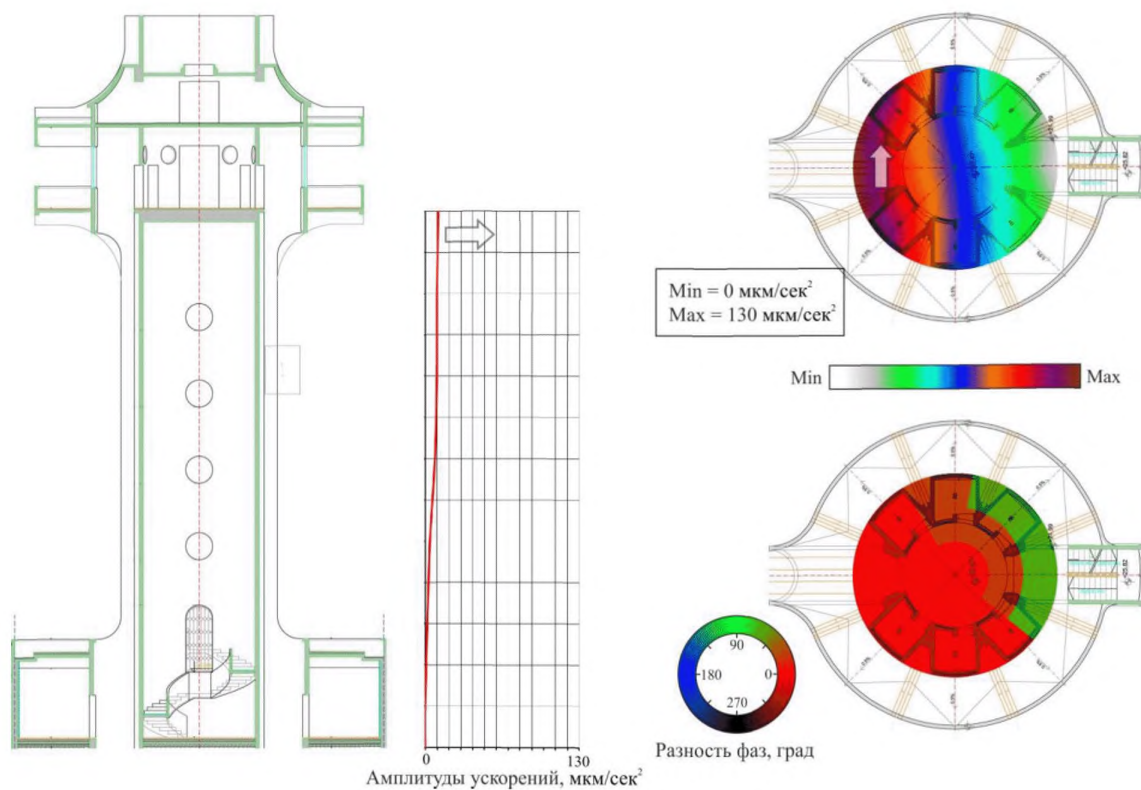
Рисунок В.11 – Пример карт амплитуд и фаз поперечного колебания
