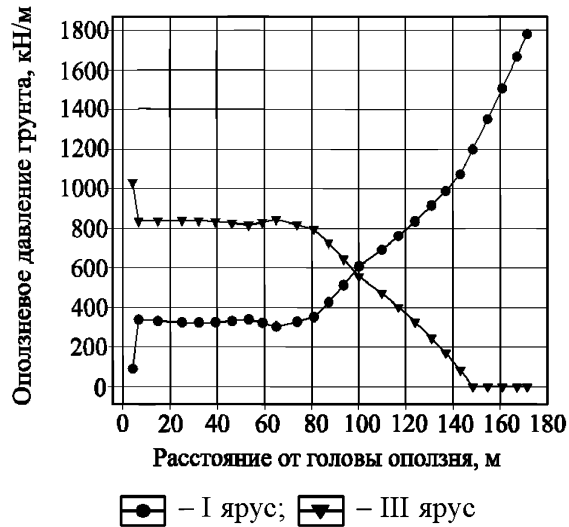
Рисунок Г.2 – Зависимость оползневых давлений в рядах от положения первого яруса (два яруса сооружений)
