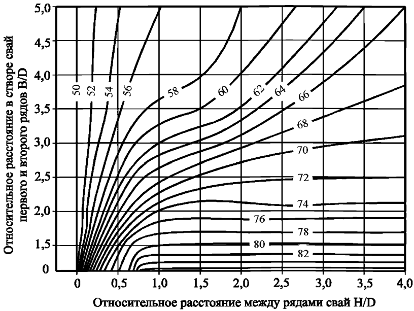
Рисунок В.17 – Номограмма для определения доли оползневой нагрузки на сваи первого ряда, % ( \bar{\alpha} = 20^\circ , \square = 0,6 )
