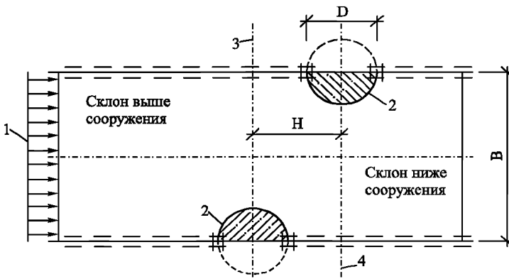
1 – оползневая нагрузка; 2 – свая; 3, 4 – оси свай соответственно первого и второго рядов; D – диаметр круглой свай; B – расстояние в створе свай первого и второго рядов; H – расстояние между рядами свай Рисунок А.1 – Расчетная схема взаимодействия грунта со сваями двухрядного удерживающего сооружения (шахматное расположение свай)
