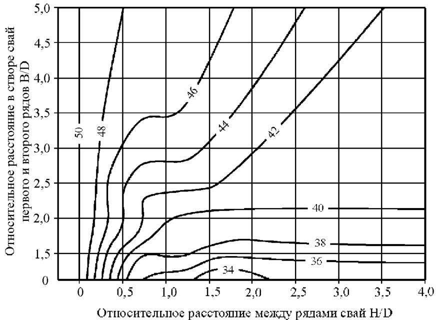
Рисунок В.4 – Номограмма для определения доли оползневой давления на сваи второго ряда, % ( \bar{\alpha} = 2,5^\circ , \square = 0,6 )
