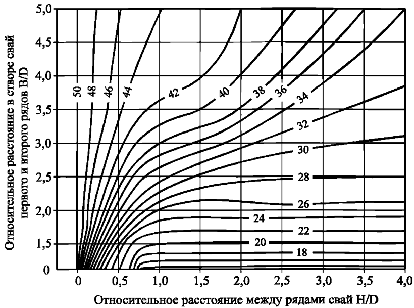
Рисунок В.18 – Номограмма для определения доли оползневой нагрузки на сваи второго ряда, % ( \bar{\alpha} = 20^\circ , \square = 0,6 )
