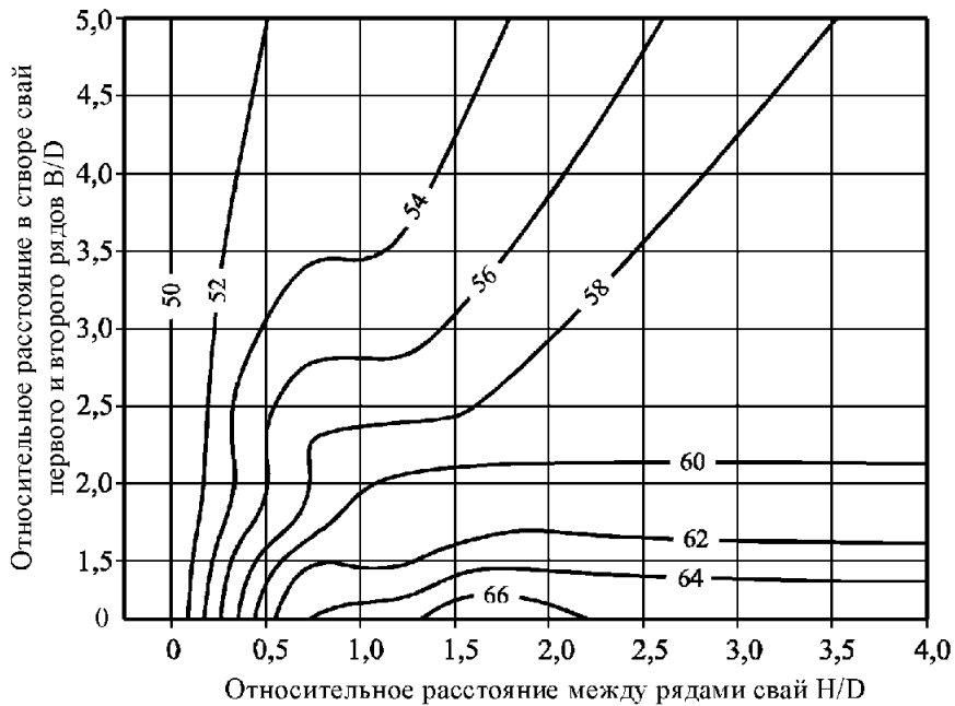
Рисунок В.3 – Номограмма для определения доли оползневой давления на сваи первого ряда, % ( \bar{\alpha} = 2,5^\circ , \square = 0,6 )
