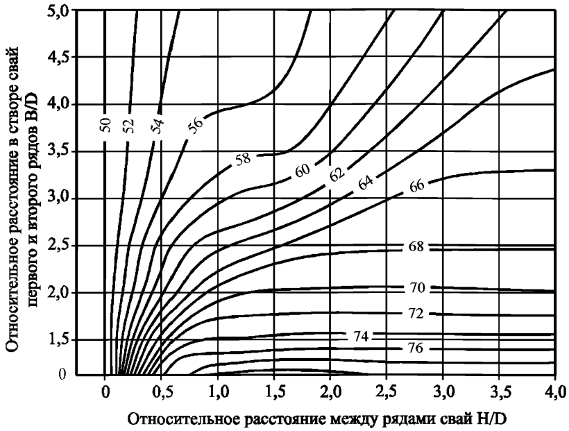
Рисунок В.13 – Номограмма для определения доли оползневого давления на
