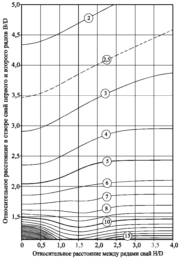
Рисунок Б.5 – Номограмма для определения удельного сопротивления свайного поля продавливаю грунту ( c = 1 кПа, \bar{\alpha} = 10^\circ , \square = 0,6 )
