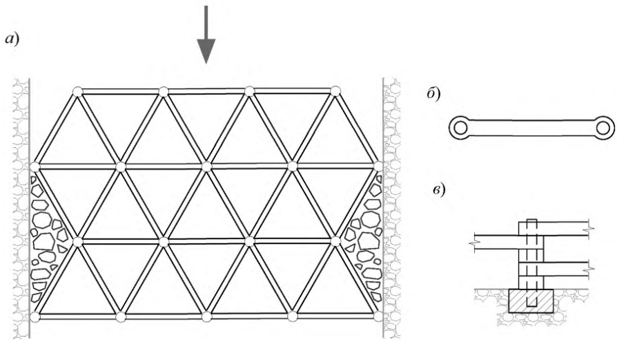
а – общий вид в плане; б – стержневой элемент; в – узел соединения элементов Рисунок 2 – Жесткое сквозное селезащитное сооружение из стержневых элементов
