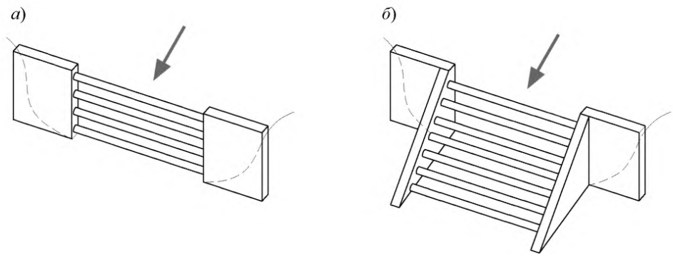
а – с вертикальной решеткой; б – с наклонной решеткой Рисунок 3 – Жесткое сквозное комбинированное селезащитное сооружение
