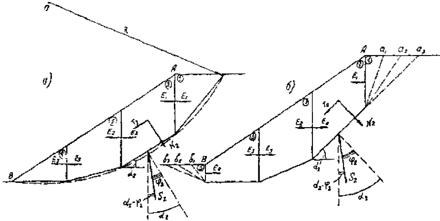
Р и с у н о к 3 – Расчетная схема к определению устойчивости по методу профессора Г.М. Шахунянца: а – поверхность скольжения проходит через подошву откоса; б – поверхность скольжения проходит через основание откоса
