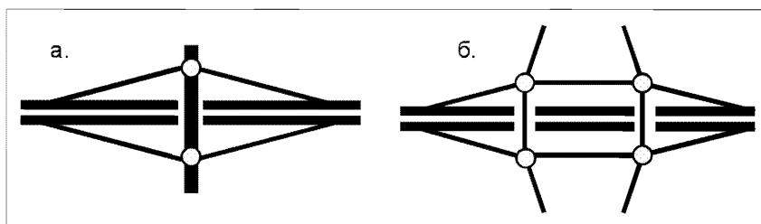
Рисунок 7.2 - Схема размещения кольцевых пересечений на второстепенном направлении транспортной развязки «неполный клеверный лист» [14]
