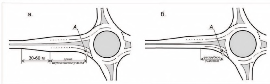
Рисунок 5.17 - Участок въезда параллельного (а) и раструбного (б) типа
