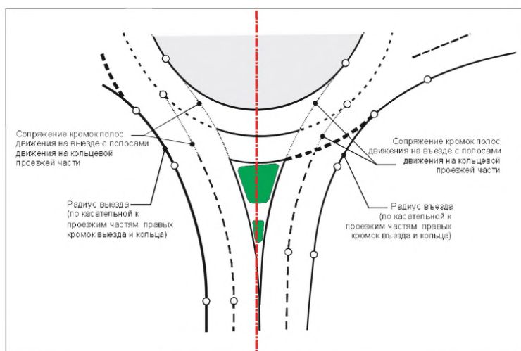
Рисунок 5.22 - Схема сопряжения кромок полос движения участка въезда – въезда с кромками полос движения кольцевой проезжей части двухполосного кольцевого пересечения
