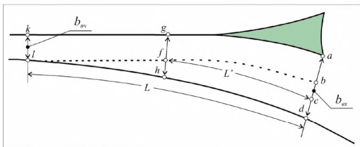
Рисунок 5.18 - Схема определения геометрических размеров раструбного упирения проезжей части на участке въезда
