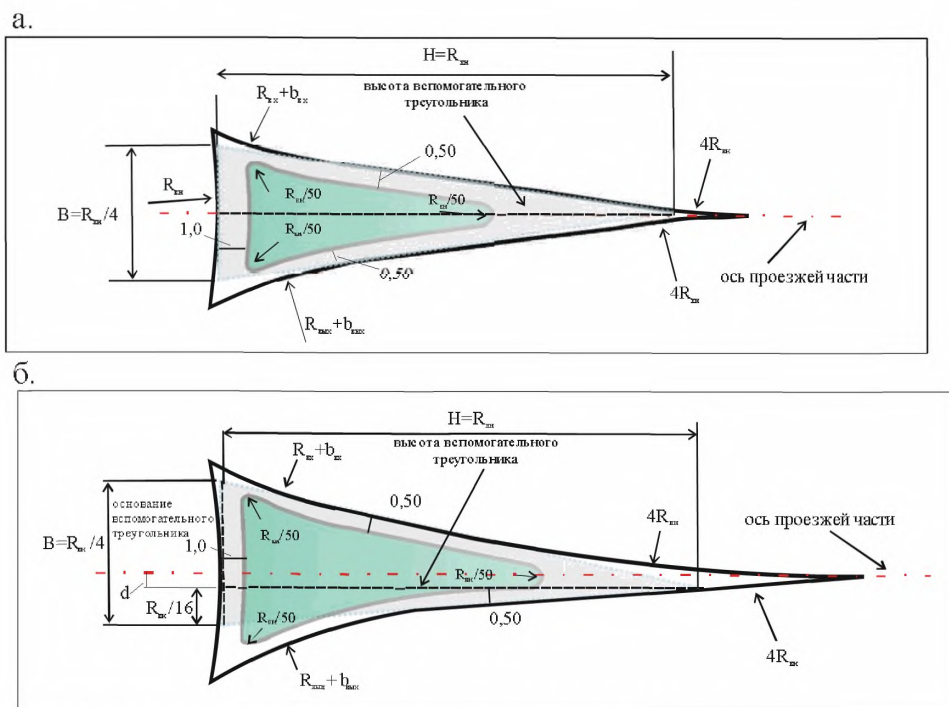
Рисунок 6.2 – Схема смещения направляющего островка на подходе к кольцевой проезжей части при радиусе внешней кромки кольцевой проезжей части ( R_{вн} ) до 15 м (а) и при радиусе внешней кромки кольцевой проезжей части свыше 15 м (б) [9]
