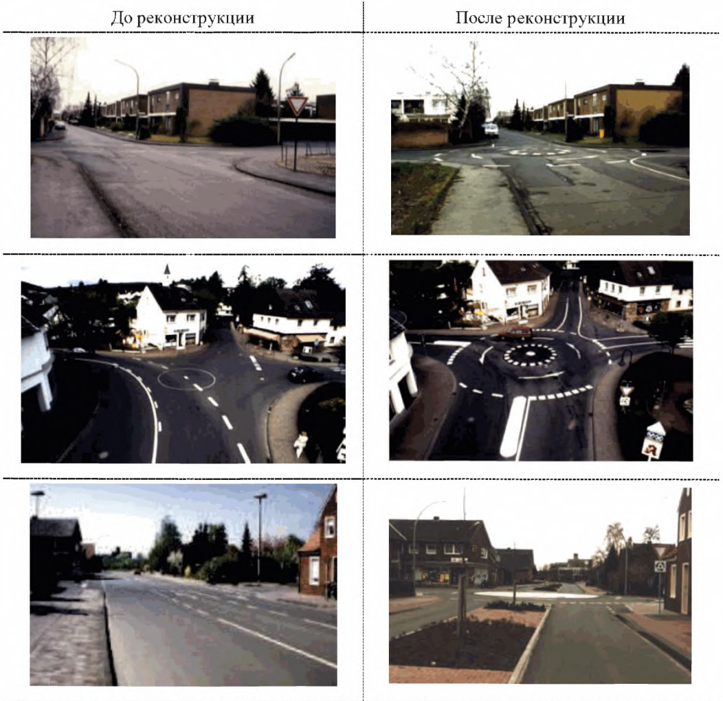
Рисунок Б.1 - Нерегулируемые пересечения (слева) и организация кольцевого движения после реконструкции [13]
