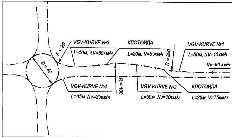
Рисунок А.1 - Проектирование основных элементов кольцевого пересечения и подходов к нему
