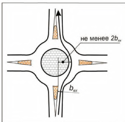
Рисунок 6.7 - Смещение траектории движения при проезде мини-кольцевого пересечения
