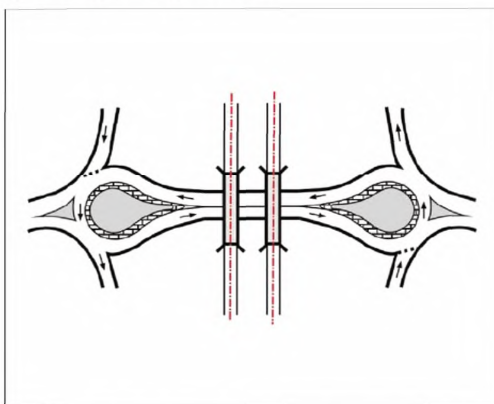
Рисунок 4.4 - Схемы основных планировочных решений кольцевых пересечений
