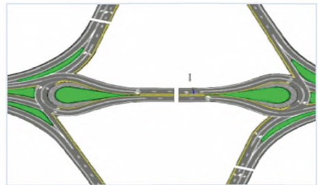
Рисунок В.2 - Кольцевая организация движения под эстакадой на второстепенном направлении [7]
