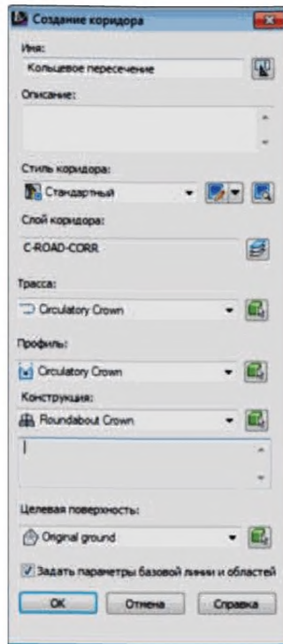
Рисунок А.20 - Диалоговое окно команды создания коридоров
