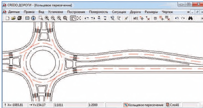
Рисунок А.4 - Кольцевое пересечение с подходами, обеспечивающими снижение скорости перед въездом на кольцо
