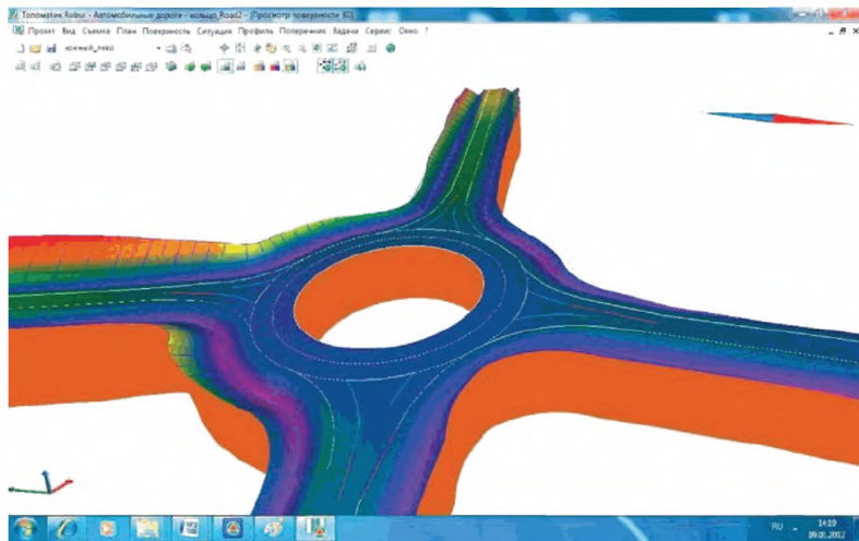
Рисунок А.13 - Комплексная проектная поверхность кольцевого пересечения
