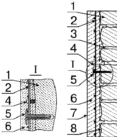
Рисунок А.16 - Восстановление кладки из кирпича или строительного камня: 1 – кладка; 2 – арматурная композитная сетка; 3 – раствор кладки; 4 – полимерный ограничитель; 5 – анкер; 6 – торкрет-бетон; 7 – поверхность после затирки; 8 – пескоструйно очищенная поверхность
