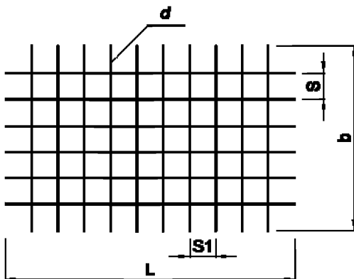
Рисунок 1 – Сетка с квадратными ячейками
