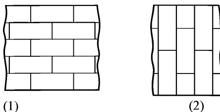
Рисунок А.2 - Варианты укладки сеток по торкретируемой поверхности: 1- укладка сеток по короткой стороне карты; 2- укладка сеток по длинной стороне карты; 3- комбинированный тип укладки карт
