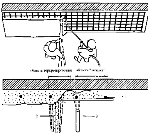
Рисунок А.9 – Удаление «отскока» сжатым воздухом:
