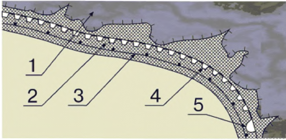
Рисунок А.12 - Поперечное сечение торкрет-бетонного покрытия с использованием в качестве водоотвода «дренажной» фольги и желоба: 1 – основание; 2- торкрет-бетон; 3 – арматурная композитная сетка; 4 – «дренажная» фольга; 5 – желоб [7]
