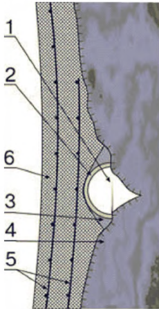
Рисунок А.12 - Поперечное сечение торкрет-бетонного покрытия с использованием в качестве водоотвода «дренажной» фольги и желоба: 1 – основание; 2- торкрет-бетон; 3 – арматурная композитная сетка; 4 – «дренажная» фольга; 5 – желоб [7]
