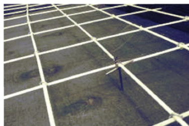
Рисунок А.1 – Общий вид стекло- и базальтокомпозитной арматуры и изготовленной из нее сетки
