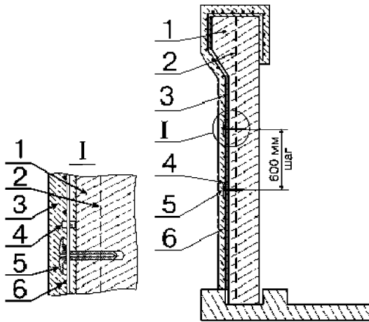
Рисунок А.17 – Подпорная стенка: 1 - усиливаемая конструкция (стена); 2 - арматура усиливаемой конструкции; 3 – торкрет-бетон усиления; 4 – полимерный ограничитель; 5 – анкер; 6 - дополнительная сетка из композитной арматуры
