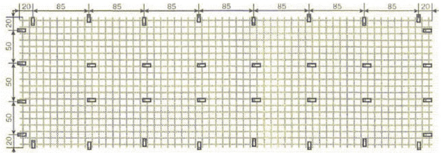
Рисунок А.3 - Схема крепления карты монтируемой сетки
