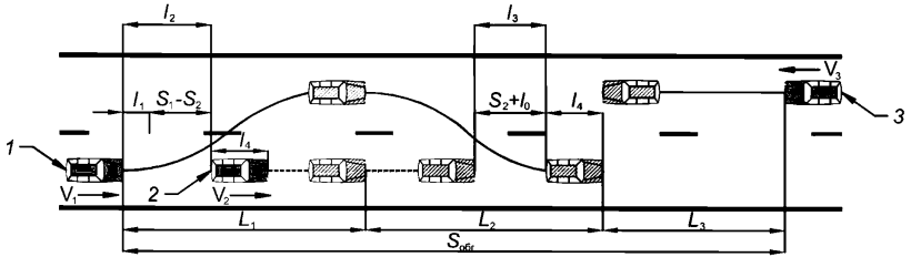
Рисунок 3 – Схема к определению расстояния видимости при обгоне
