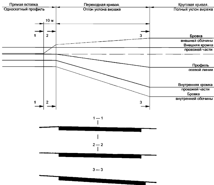
Рисунок 32 – Преобразование однокатного поперечного профиля на виражах вращением относительно внутренней кромки проезжей части
