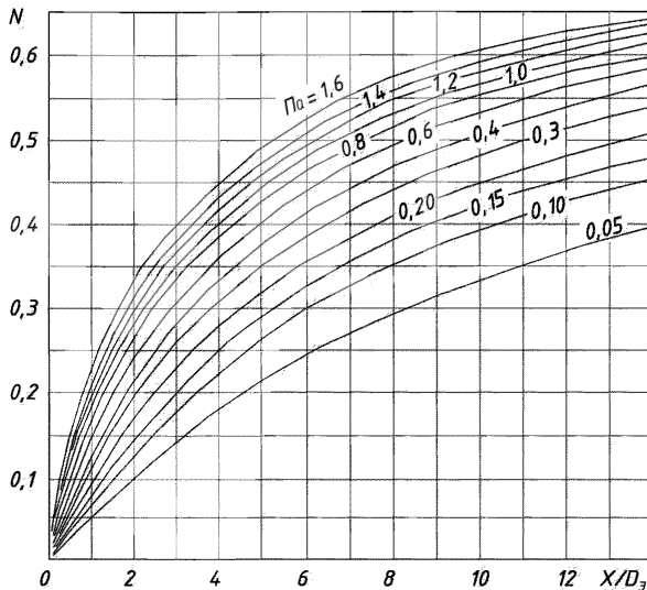
Рисунок 13 – График для определения параметра N
