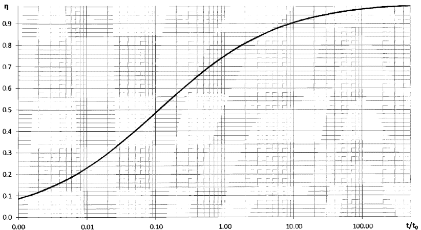
Рисунок 15 – График для определения относительной глубины размыва
