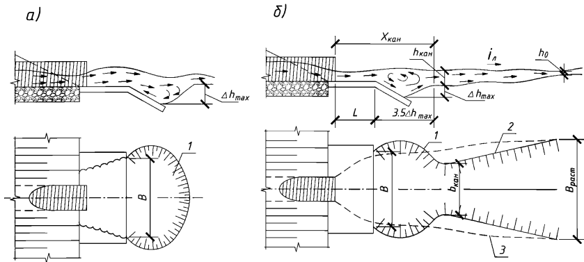
а - поверхностный; б - донный; 1 - контур воронки размыва; 2 - контур канавы; 3 - границы растекания
