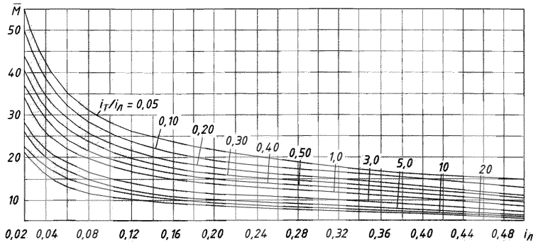
Рисунок 12 – График для определения параметра \bar{M}
