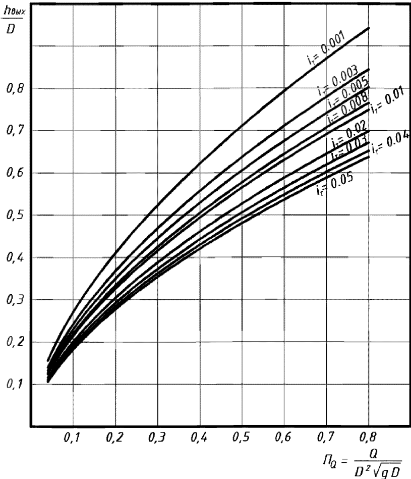
Рисунок 5 – График для определения глубины потока на выходе из трубы
