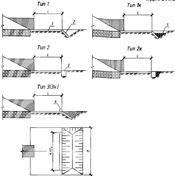
Рисунок 6 – Типы выходных русел
