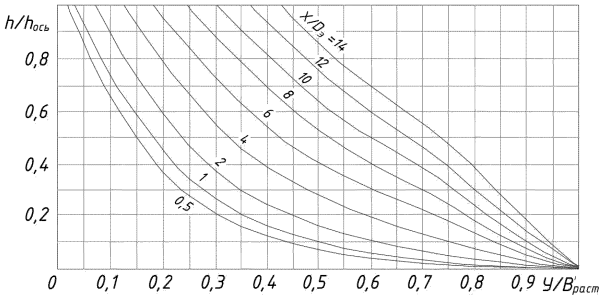
Рисунок 9 – График для определения глубины потока h на укреплении
