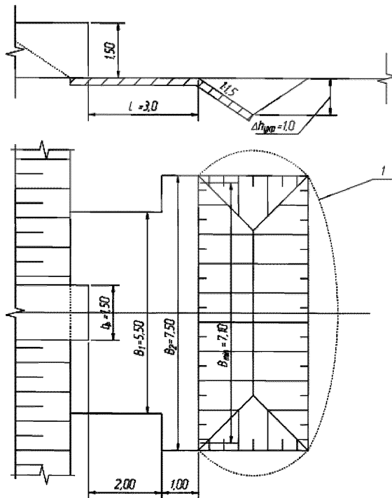
Рисунок Б.1 – Конструкция и размеры укрепления, полученные в результате расчета нижнего бьефа трубы
