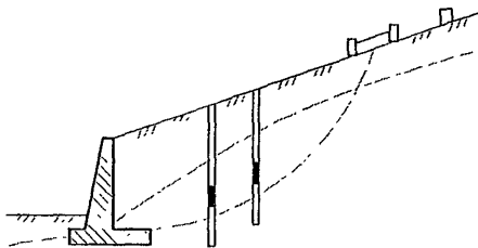
Рисунок 3 – Пример схемы расположения измерительного оборудования на оползнеопасном склоне
