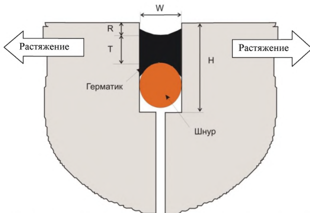
Рисунок Б.1. Схема работы герметика в сечении деформационного шва при охлаждении покрытия
