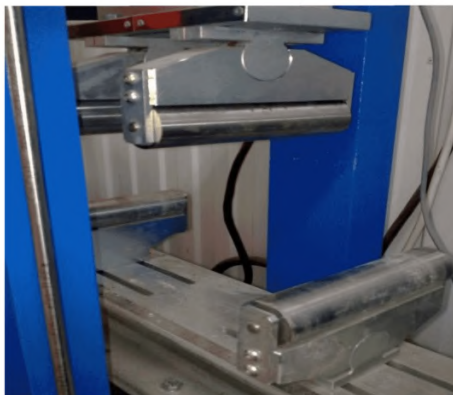
Рисунок 4.3 – Вид траверсы пресса для испытания бетона на прочность на растяжение при изгибе
