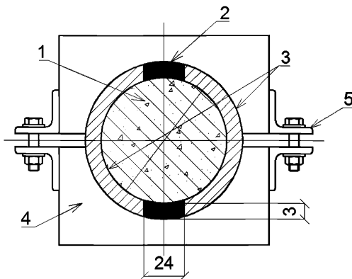
Рисунок 4.5 – Схема устройства подливки вдоль керна по двум образующим с помощью кондуктора:
