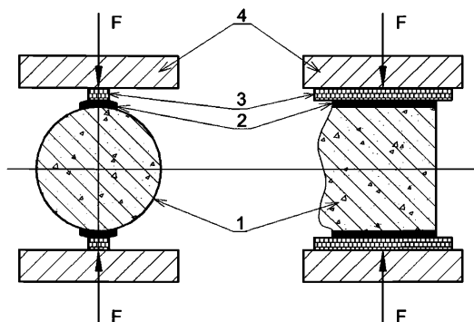
Рисунок 4.7 – Схема испытания на раскалывание керна с продольными подливками:
