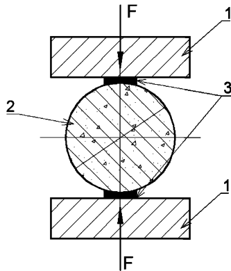
Рисунок 4.4 – Схема испытания керна на растяжение при раскалывании:
