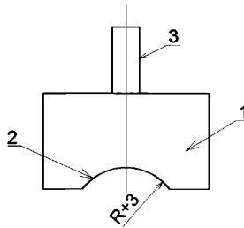
Рисунок 4.6 – Гладилка для обработки поверхности продольной подливки:
