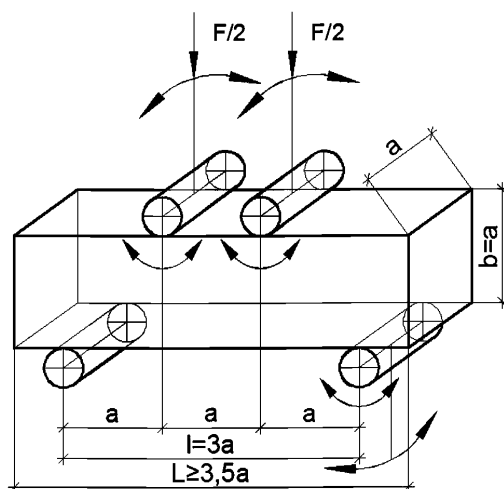
Рисунок 4.2 – Схема испытания бетона на прочность на растяжение при изгибе
