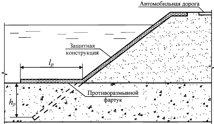
Рисунок 2 – Определение длины выпуска противоразрывной конструкции
