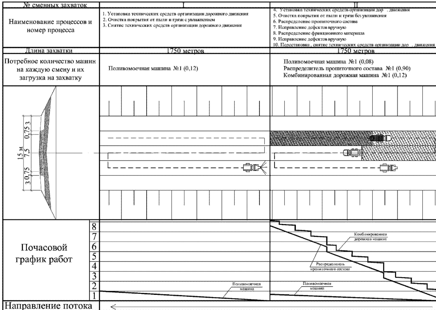
Рисунок Ж.2 – Технологический план потока по нанесению ДПМ без минерального наполнителя в составе
