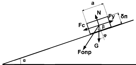
Рисунок 12 – Расчетная схема опрокидывания блока
