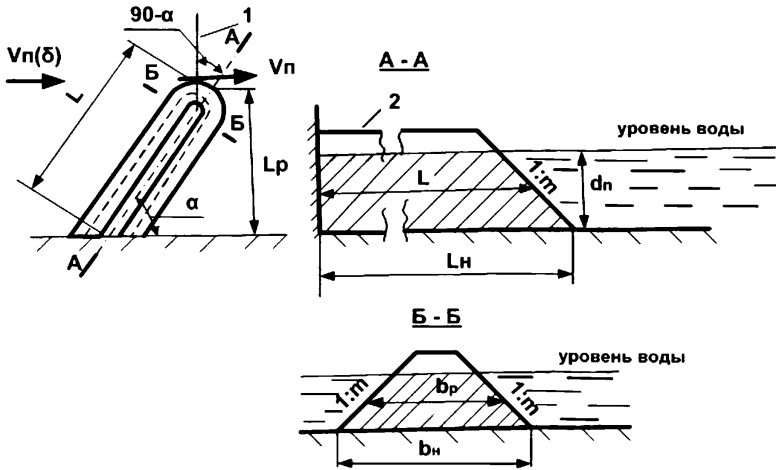
Рисунок 4 – Траверс у пойменной насыпи
