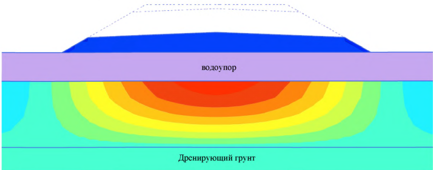
Рисунок 26 – Консолидируемый слой подстиляется дренирующим, а перекрыт водоупором (аналогично пути фильтрации «только вниз»)
