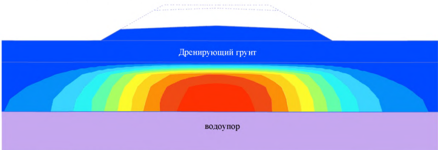
Рисунок 27 – Консолидируемый слой заключен подстиляется водоупором, а перекрыт дренирующим (аналогично пути фильтрации «только вверх»)
