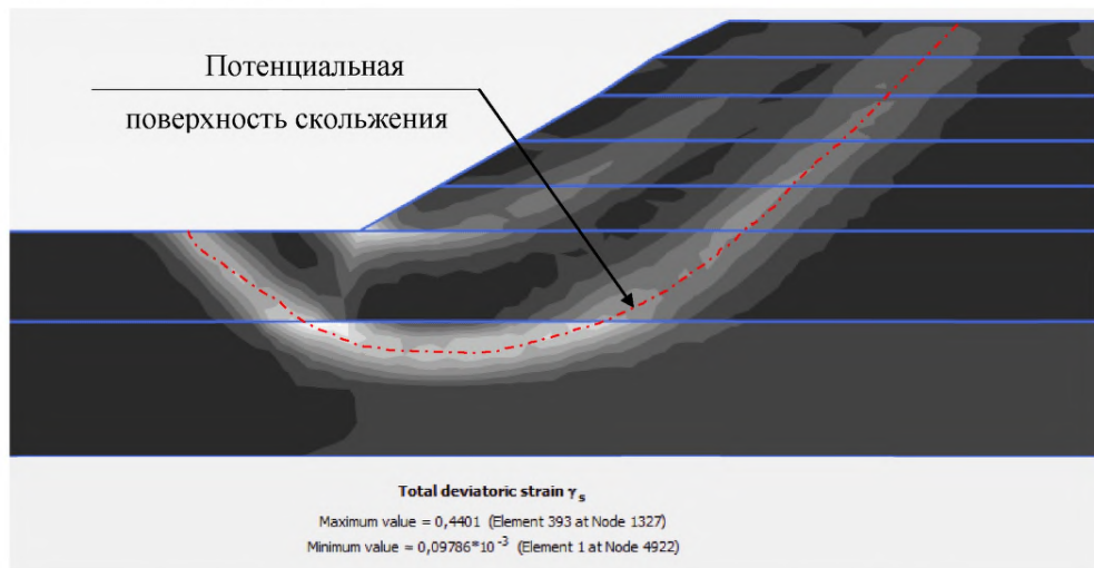
Рисунок 21 – Изополя приращения сдвиговых деформаций \Delta\gamma_s
