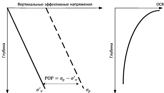
Рисунок 4 – Профиль давления предуплотнения (слева) и профиль коэффициента переплотнения OCR (справа) по глубине при использовании величины исторической нагрузки POP
