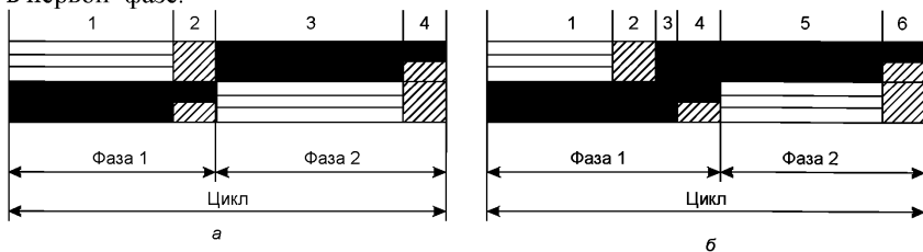
Рисунок 7 - Структура светофорного цикла:
