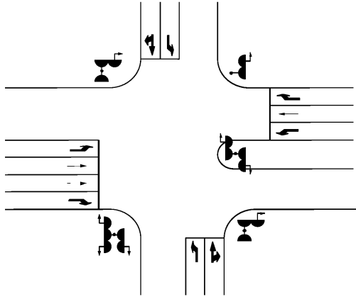
Рисунок 3 - Пример расположения в плане транспортных светофоров
