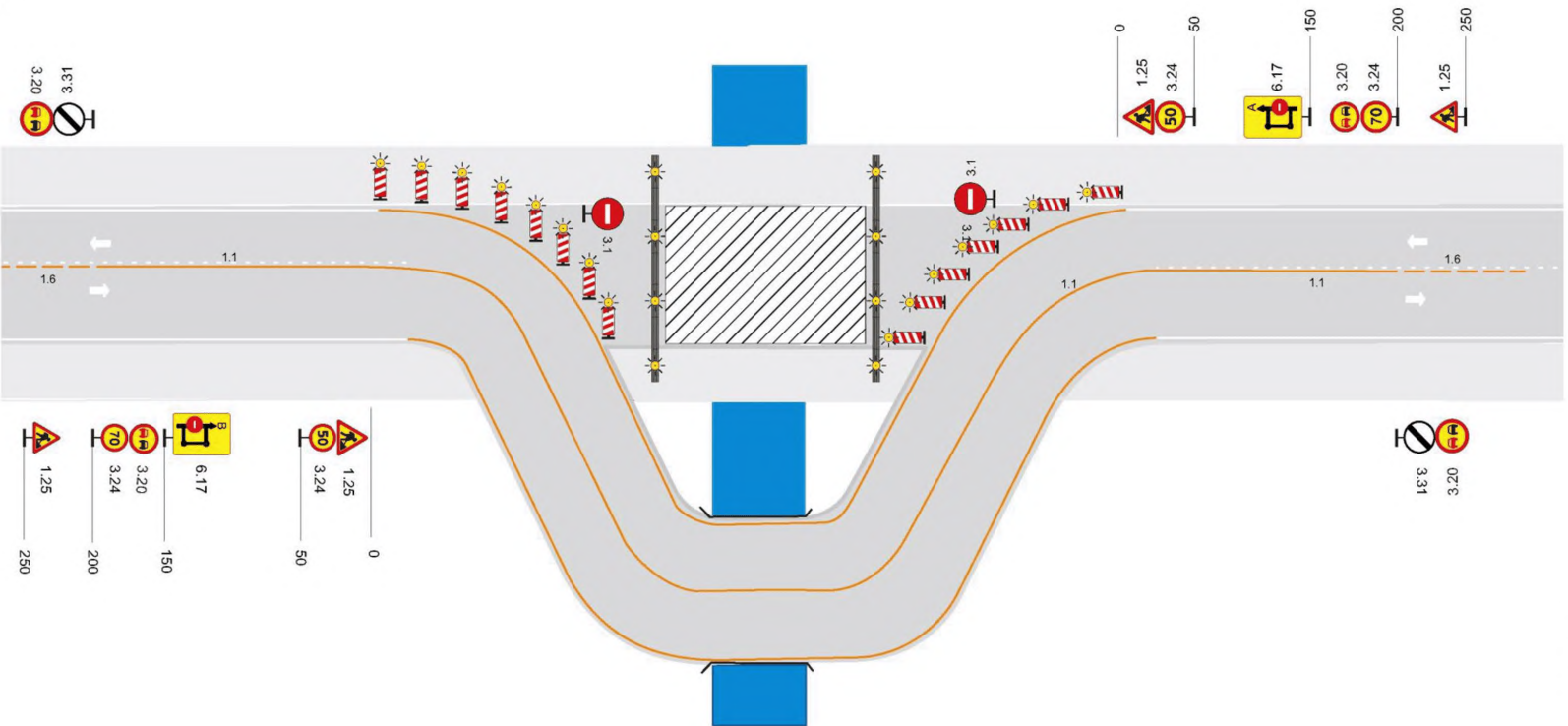
Рисунок Б.10 - Двухполосная дорога. Рабочая зона долговременных работ на мосту. Пропуск транспортных средств по специальному устройству объезду
