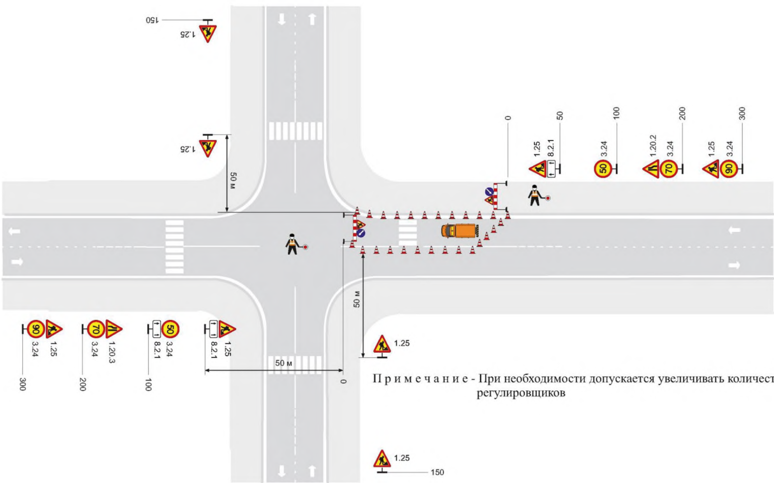
Рисунок Б.39 - Пересечение автомобильных дорог в одном уровне. Рабочая зона краткосрочных работ по нанесению дорожной разметки на полосу движения. Пропуск транспортных средств по полосе встречного движения с помощью регулировщиков
