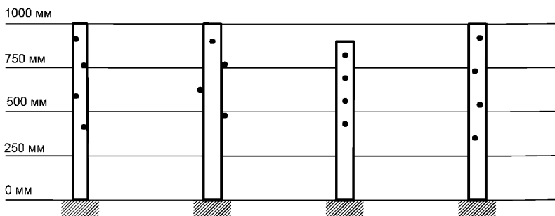
Рисунок 3 – Расположение тросов по высоте отечественных конструкций
