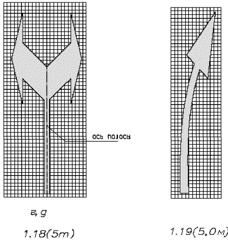
Рисунок Б.1 - Схемы дорожной разметки 1.18 и 1.19 длиной 5,0 м
