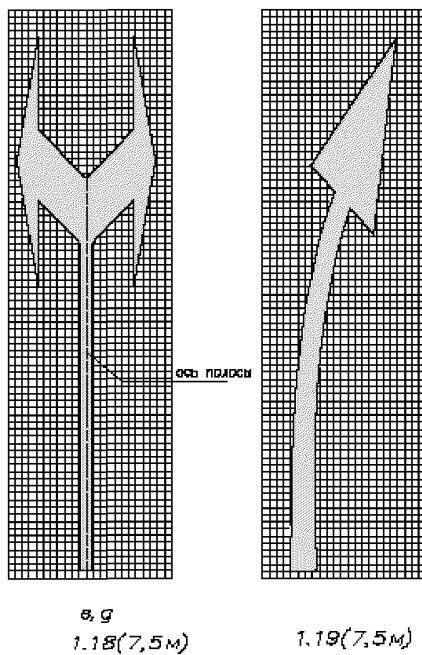
Рисунок Б.2 - Схемы дорожной разметки 1.18 и 1.19 длиной 7,5 м
