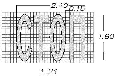
Рисунок Б.3 - Схемы дорожной разметки 1.20 и 1.21
