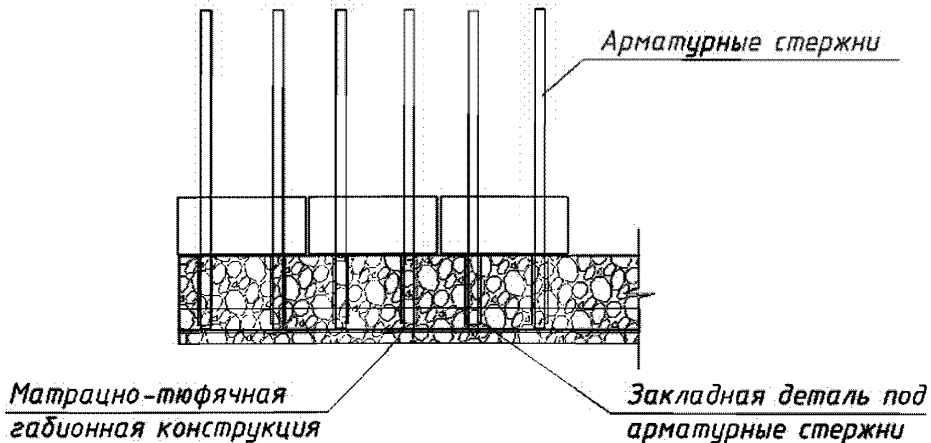
Рисунок Ж.4 – Установка первого ряда блоков
