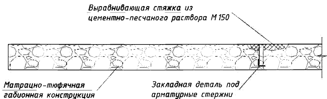
Рисунок Ж.3 – Установка закладной детали в матрацно-тюфячную габионную конструкцию
