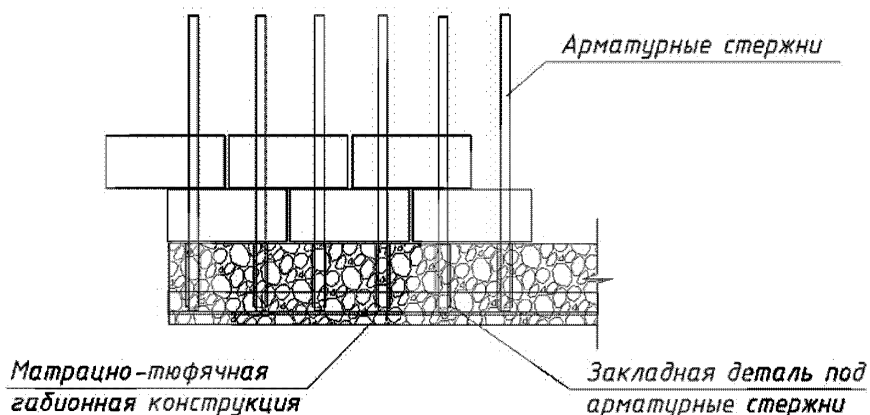
Рисунок Ж.5 – Установка второго ряда блоков
