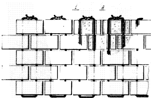
Рисунок 7 – Схема модульного блока ГПП
