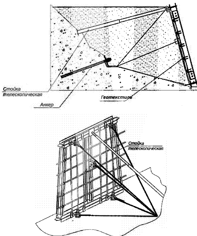
Рисунок 6 – Конструкция зонтичного сооружения на тросах
