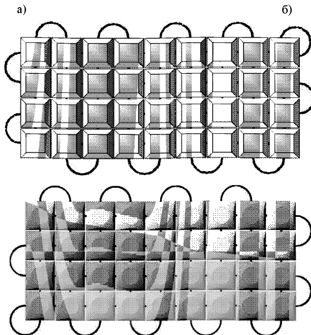
а), б) – варианты бетонных блоков КГПП в), г) – маты КГПП из представленных выше блоков, соответственно
