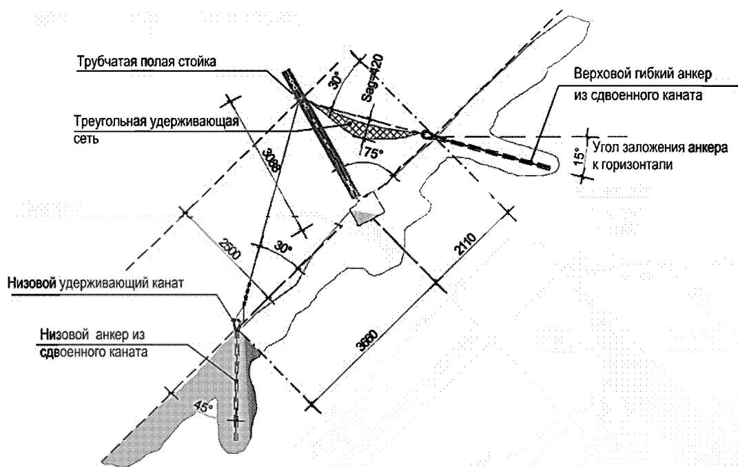
Рисунок К.1 – Поперечное сечение снегозадерживающего ограждения
