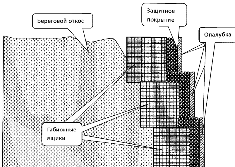
Рисунок 20 – Защита ступенчатой габрионной стены
