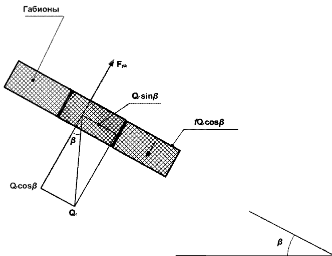
Рисунок 14 – К расчету устойчивости габионов на откосе
