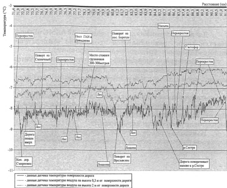
Рисунок Г.2. Вид первичной, расшифрованной термокарты (термофиль)
